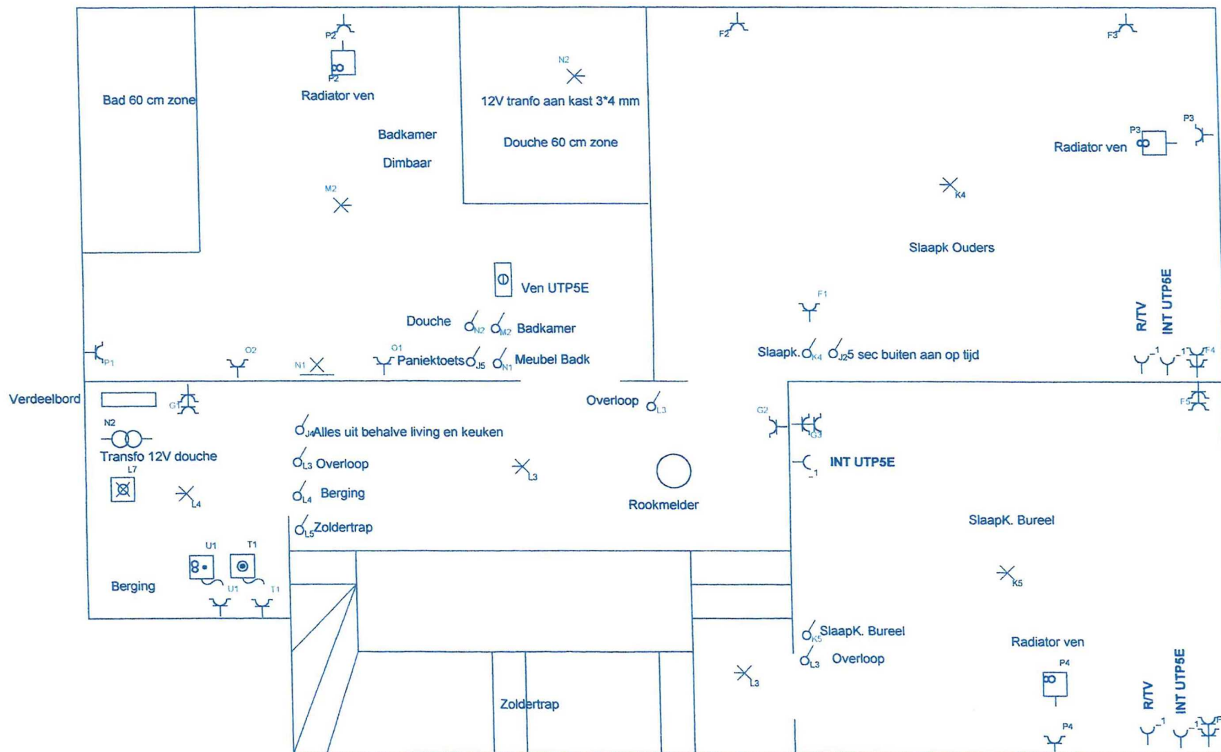
Situatieschema 1 ste verdiep slaapk.
